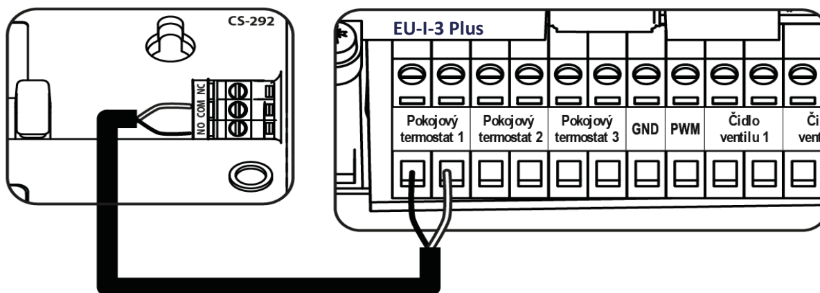
Příklad zapojení dvupolohového (ON/OFF) termostatu
